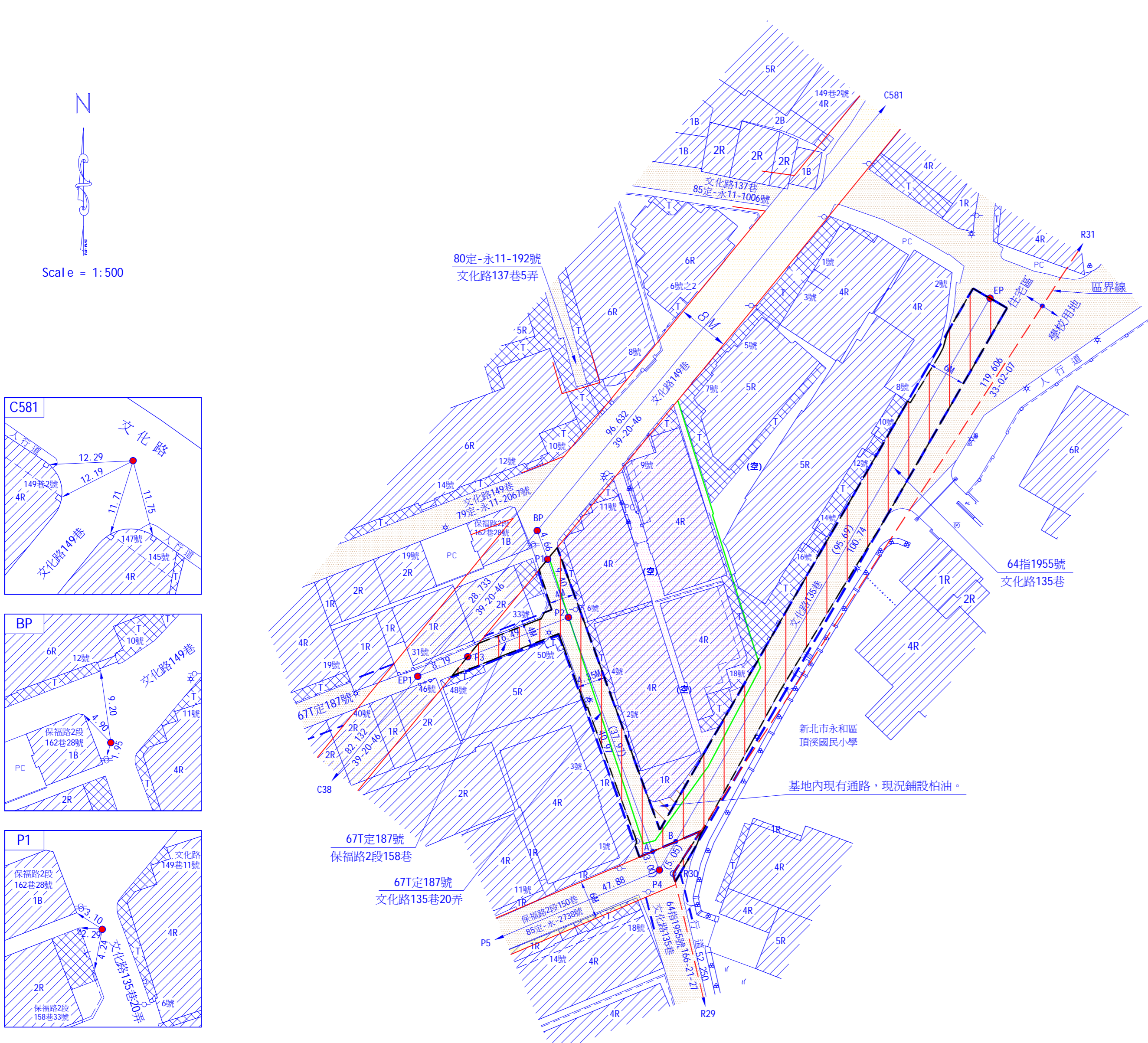
現況計畫圖 SCALE 1/500
