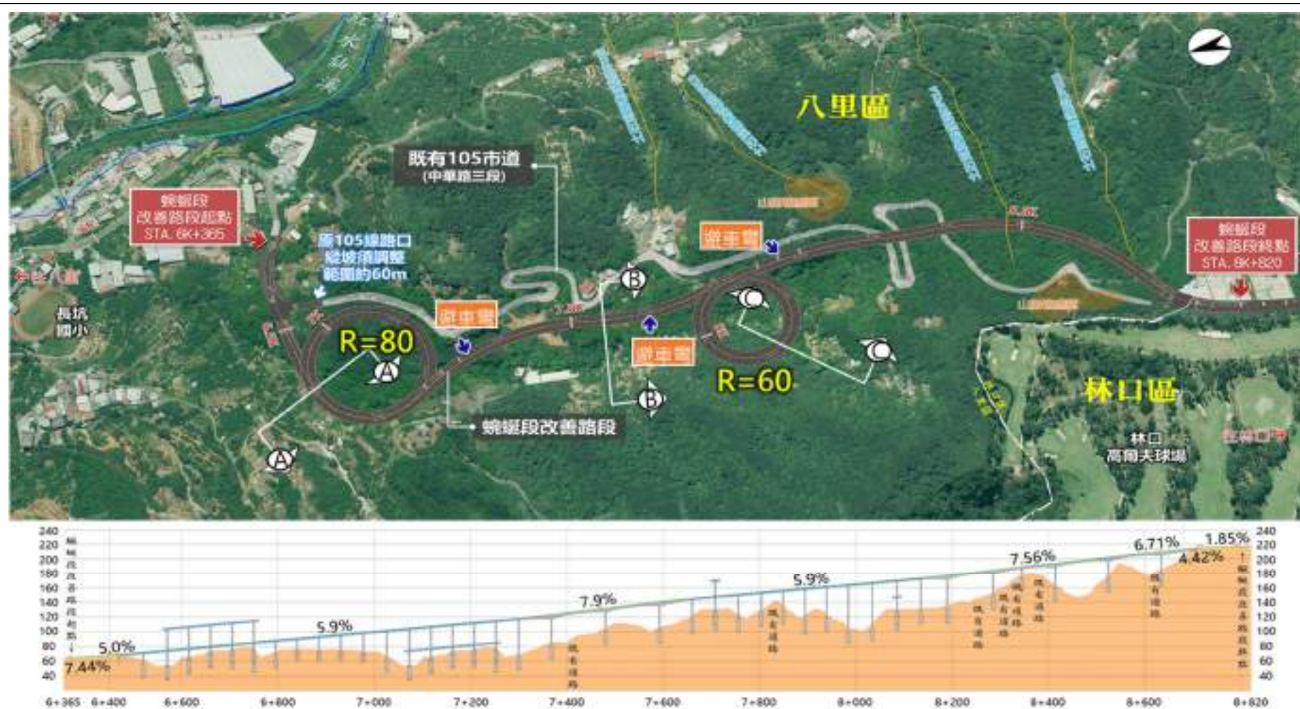
圖13 本案路段路線平、縱面示意圖
