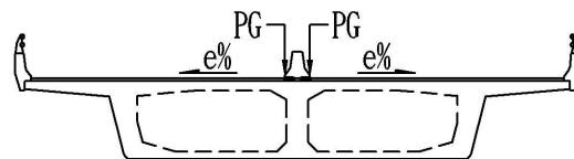
断面 B 新闢道路 一般路段
