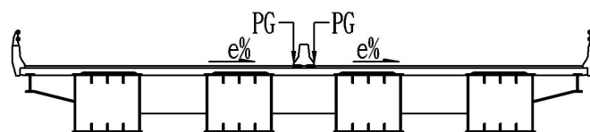
断面 C 新闢道路 南端環橋(R=60M)
