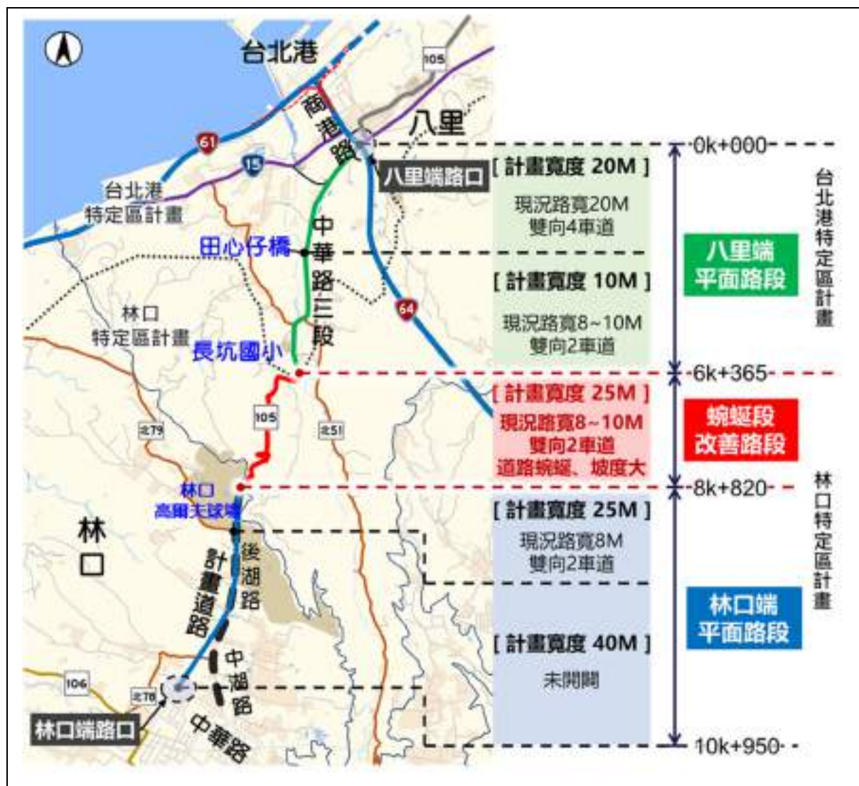
圖1 本計畫路段分段示意圖
